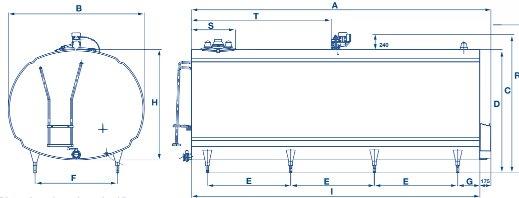
Dimensioner i mm; kapacitet i liter
