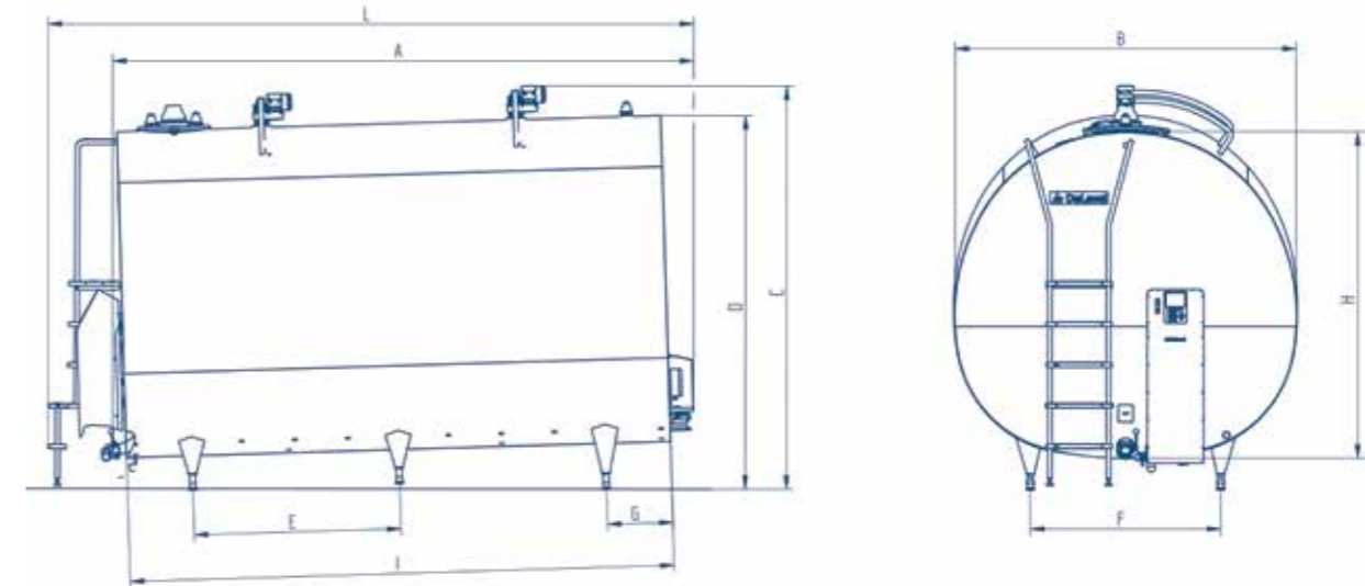
Dimensioner i millimeter
